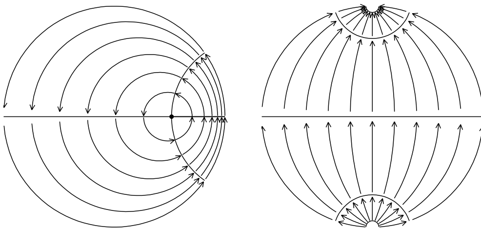
OBRÁZEK 5. Rotace PLHP (vlevo) a posun HPLP (vpravo)
