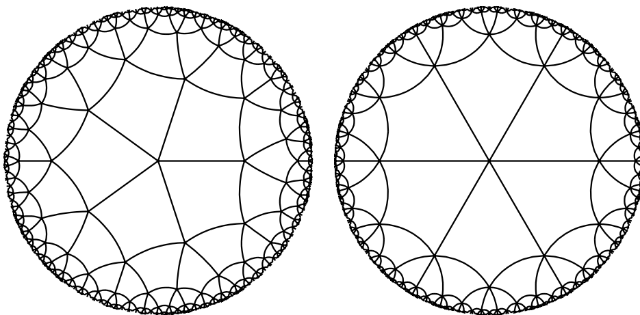
OBRÁZEK 3. Čtvercové teselace hyperbolické roviny: n = 4 , m = 5 (vlevo), m = 6 (vpravo)
