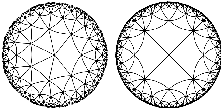
OBRÁZEK 2. Trojúhelníkové teselace hyperbolické roviny: n = 3 , m = 7 (vlevo), m = 8 (vpravo).
