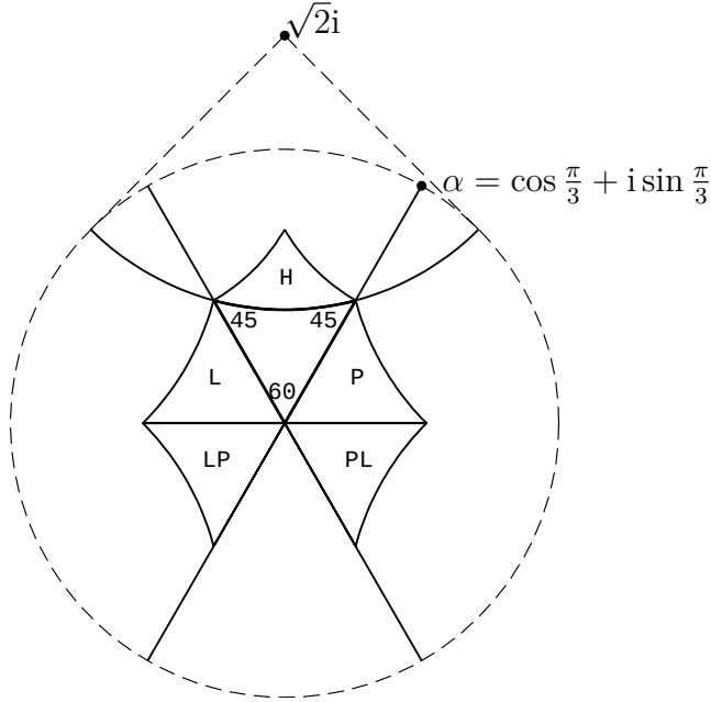
OBRÁZEK 4. Reflexe rovnoramenného trojúhelníka
